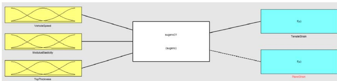
شکل ۶. مدل پیش‌بینی خرابی بحرانی روسازی انعطاف‌پذیر مبتنی بر سرعت وسیله نقلیه در محیط متلب
