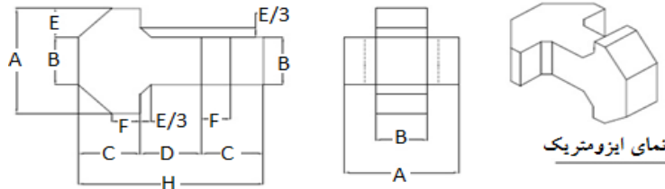
شکل ۸. ابعاد و پارامترهای طراحی توسکان‌ها
