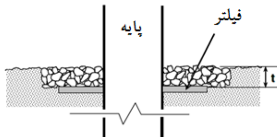
شکل ۱. ضخامت سنگچین اطراف پایه
