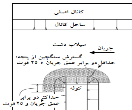
شکل ۳. پلان امتداد پیشبند سنگچین اطراف کوله
