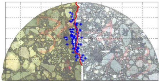
شکل 6. نحوه تعیین مکان ترک به روش AE روی سطح نمونه
