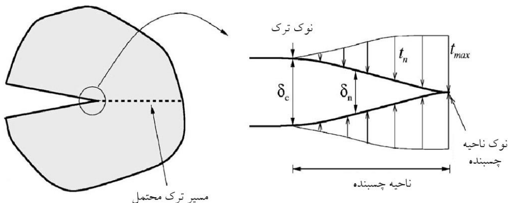
شکل 3. نمایش شماتیک مفهوم ناحیه چسبنده (Song, Paulino and Buttlar, 2006)
