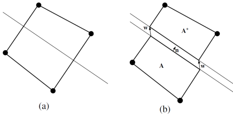
شکل 4. یک المان محدود با ترکی به صورت بازشدگی یکنواخت: (a) بدون ترک خوردگی و (b) با پرش تغییر مکان یکنواخت در راستای خط ترک (Wu, Denneman and Harvey, 2009)
