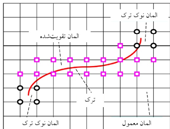
شکل 5. نمایش گره‌های تقویت شده در XFEM (Wang et al., 2013)
