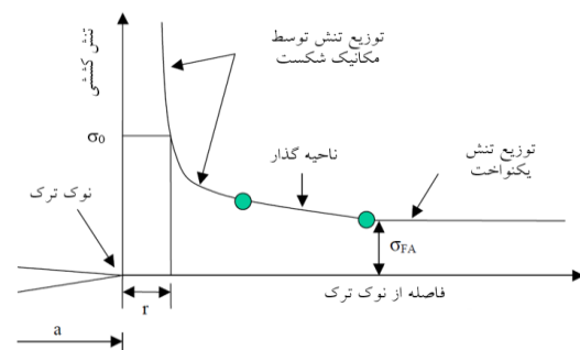
شکل 2. توزیع تنش در جلوی نوک ترک (Sangpetngam, Birgisson and Roque, 2003)
