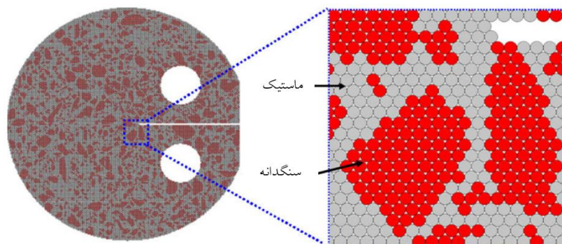
شکل 7. مش نمونه المان گسسته (DEM) با آرایش شش ضلعی (Kim, Buttlar, 2009)
