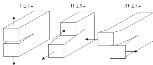
شکل 1. حالات تنش ترک ها (Mojiri, 2010)
