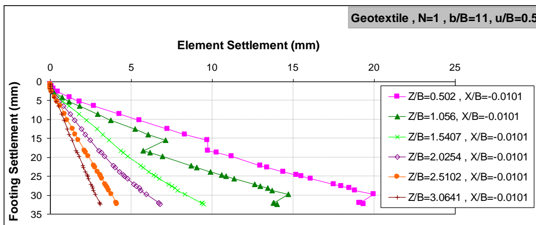
شکل 10. نمودار نشست پی - نشست المانهای خاک در Z/B های مختلف (Test 5)
