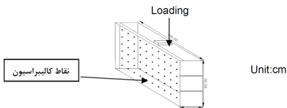
شکل 3. جعبه آزمایش
