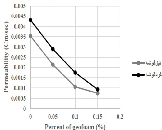
شکل ۱۲. تاثیر ذرات ژئوفوم بر میزان نفوذ پذیری مصالح مورد استفاده (توفیق آذری و دبیری، ۱۳۹۷)
