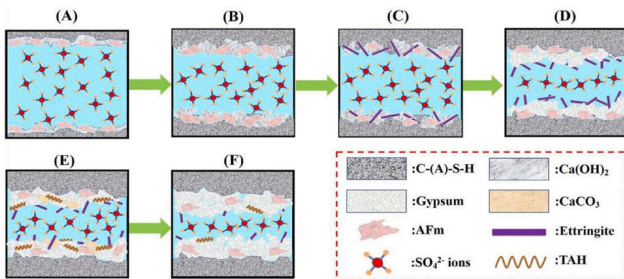
شکل ۱۰. تغییرات مورفولوژیکی در ترکیب فازی محصولات خوردگی در هنگام حمله سولفات در مقادیر pH پایین (G. Zhang et al., 2021)
