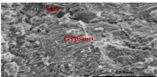
(c) ۲۸ روز، pH=8
