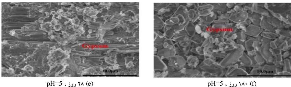
شکل ۹. مورفولوژی گچ و اترینگیت در خمیر سیمان پرتلند در معرض حمله سولفات در مقادیر مختلف pH (G. Zhang et al., 2021)
