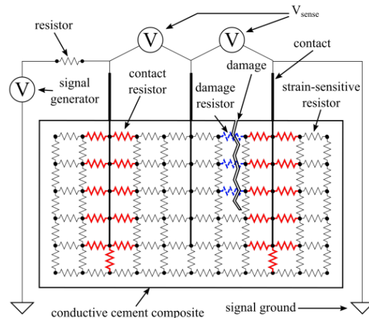
شکل ۷. شماتیک از مدل مش مقاومت
