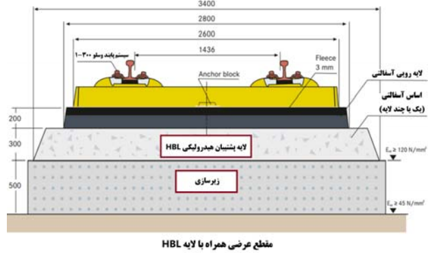
شکل ۱۱. مقطع متداول خطوط گترک از نوع A1 همراه با لایه پشتیبان هیدرولیکی (Yang, Wang, Qiu et al. 2016)
