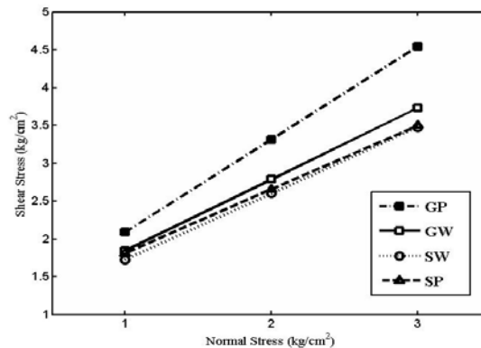
شکل ۳. مقایسه پوش‌های گسیختگی برای ۴ نوع مصالح
