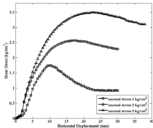
شکل ۵. نمودارهای تنش برشی در مقابل جابجایی برشی برای ماسه SW برای سه سربار مختلف
