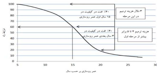
شکل ۱. ارتباط هزینه‌های ترمیم و نگهداری با افزایش عمر روسازی (هاشمی، ۱۳۹۵)
