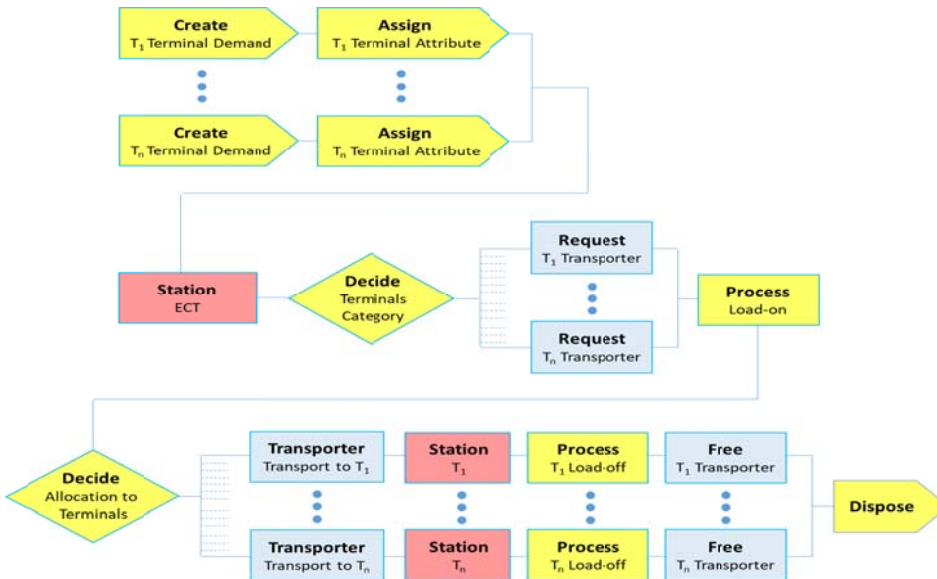
شکل ۲. فلوچارت عملیات تخصیص کانتینرهای خالی
