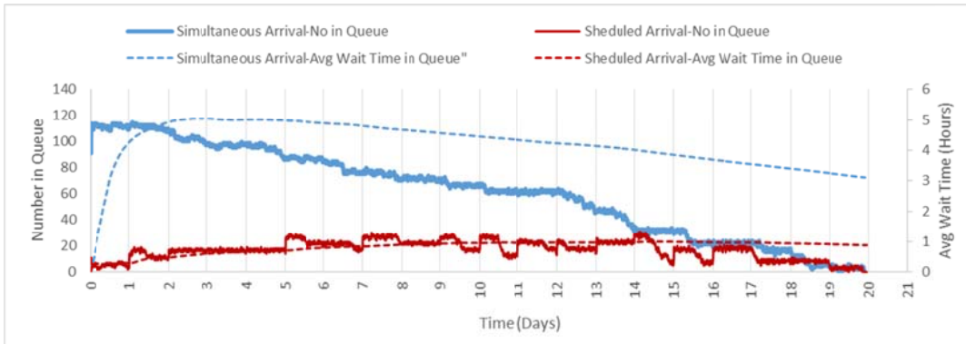
شکل ۶. مقایسه صف بارگیری در دو حالت فراخوانی همزمان / غیرهمزمان کشنده‌ها- سناریوی اصلاح تقاضا
