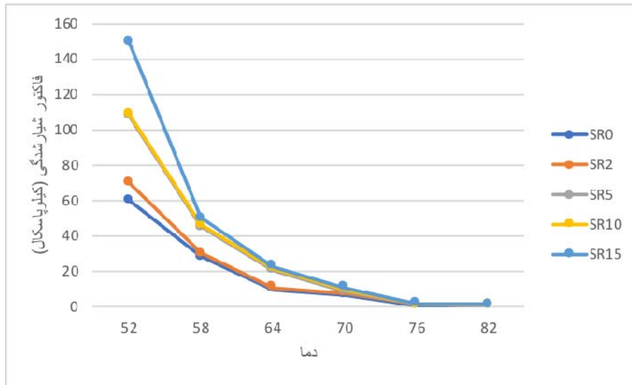
شکل ۹. فاکتور شیارشدگی: الف) پیرنشد. ب) پیرشده (ب)
