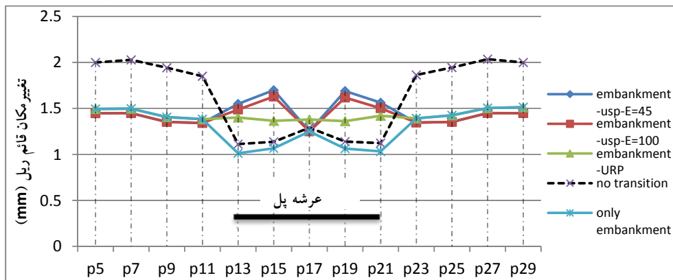
شکل ۱۶. تغییر مکان قائم ریل برای حالت‌های مختلف روش انتقال سختی ترکیبی
